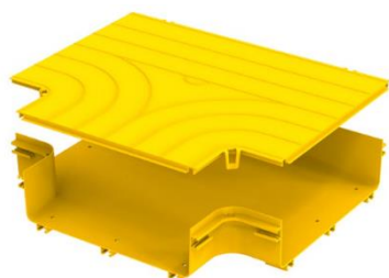
Horizontal Tee
